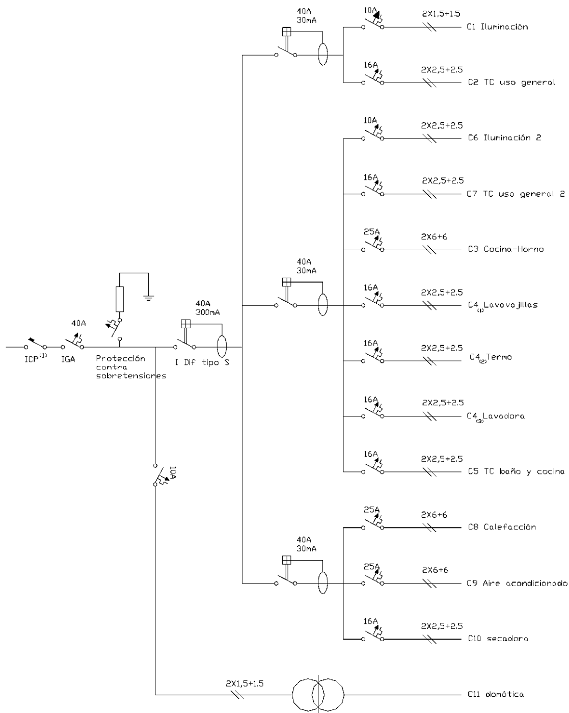
Fig. 20: Ejemplo de esquema unifilar de una vivienda con electrificación elevada (Fuente: GUIA-BT-25 [5])
