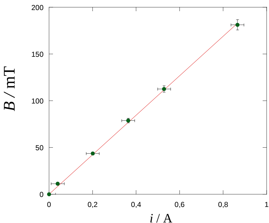
Figura 1. Valor experimental del campo magnético en el interior del solenoide en función de la intensidad de corriente que circula por él. Se ha realizado un ajuste a una recta cuya ecuación es B = (211.2 \pm 1.7) i expresando la pendiente en mT/A.
