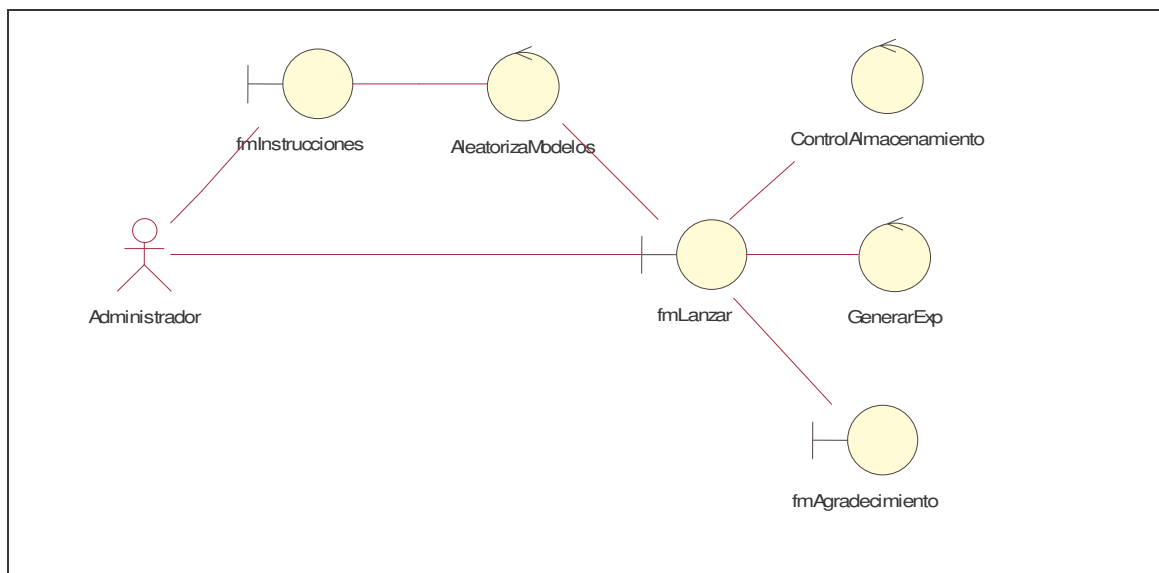
Figura A.17. Clases del caso de uso-análisis Simular Encuesta o Experimento
