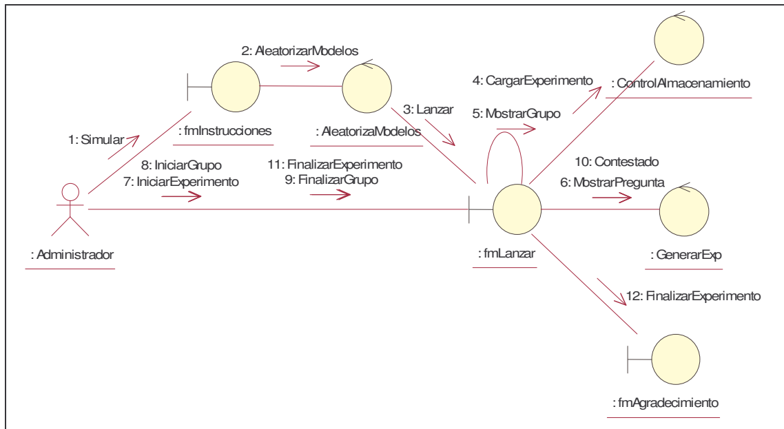
Figura A.18. Interacción de las clases para el caso de uso Simular Encuesta o Experimento
