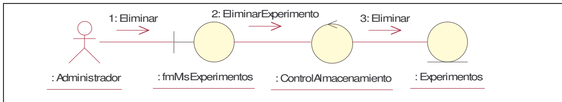
Figura A.14. Interacción de las clases para el caso de uso Eliminar Encuesta o Experimento
