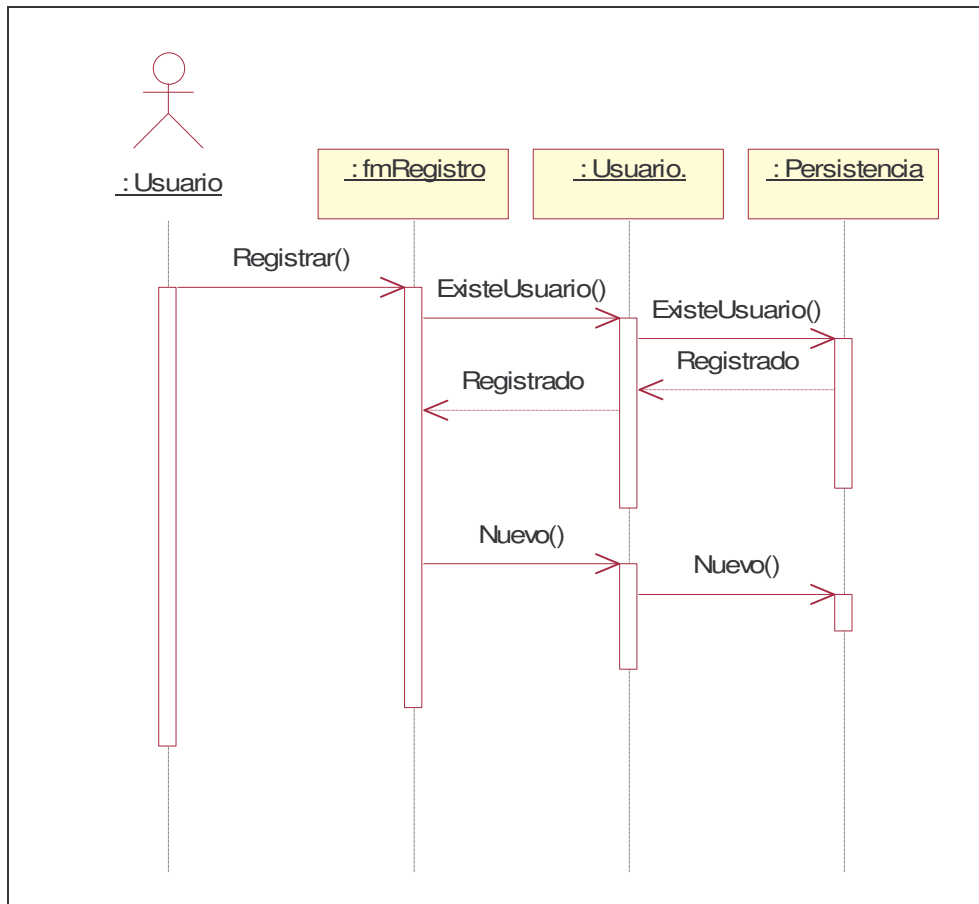
Figura A.8. Diagrama de Secuencia del caso de uso Registrarse
