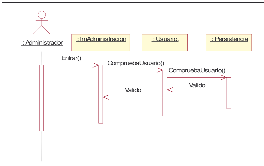
Figura A.4. Diagrama de Secuencia del caso de uso Autenticar
