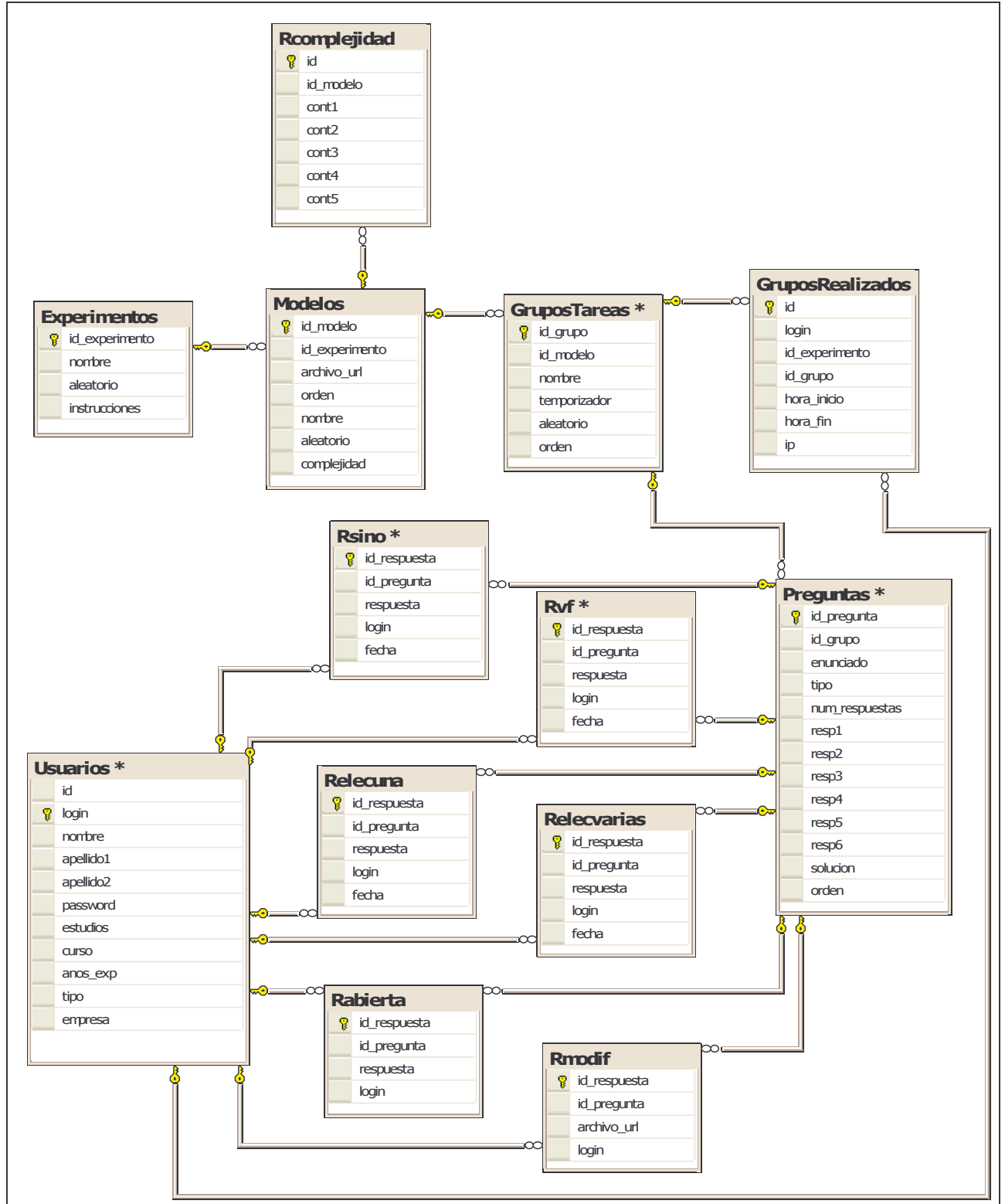
Figura 5.16. Base de datos Empirical-WebGen
