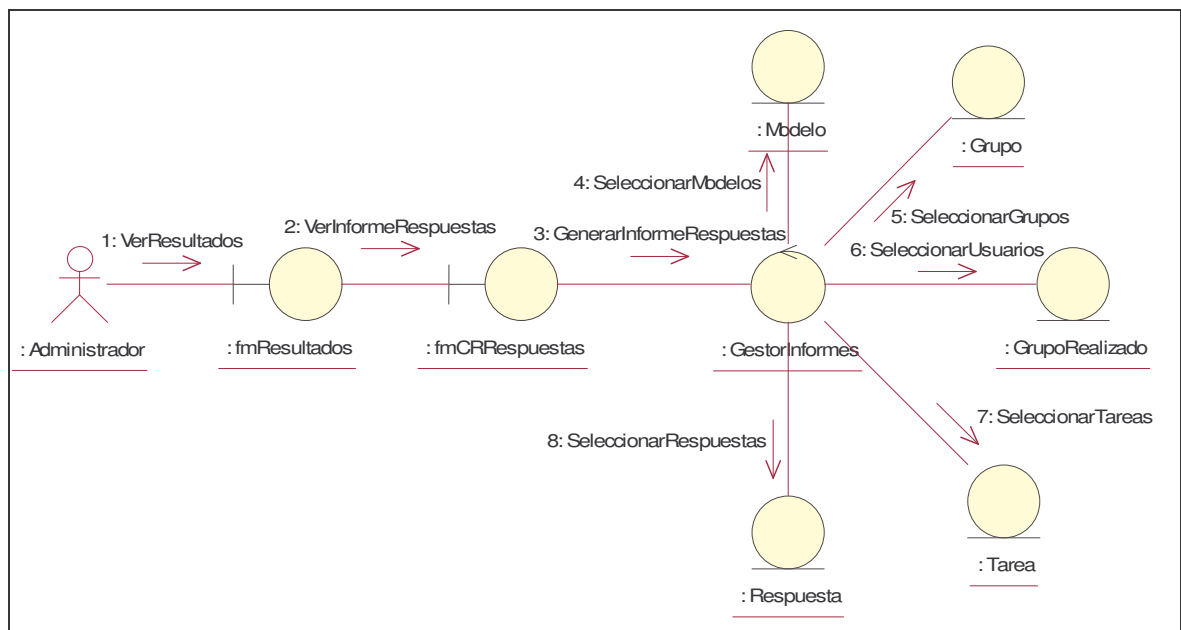
Figura A.22. Interacción de las clases para el caso de uso Visualizar Respuestas
