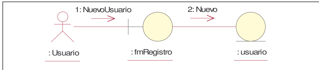
Figura A.6. Interacción de las clases para el caso de uso Registrarse
