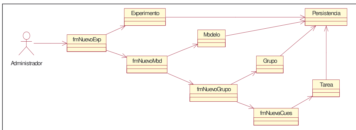
Figura 5.9. Clases del caso de uso-diseño Definir Encuesta o Experimento
