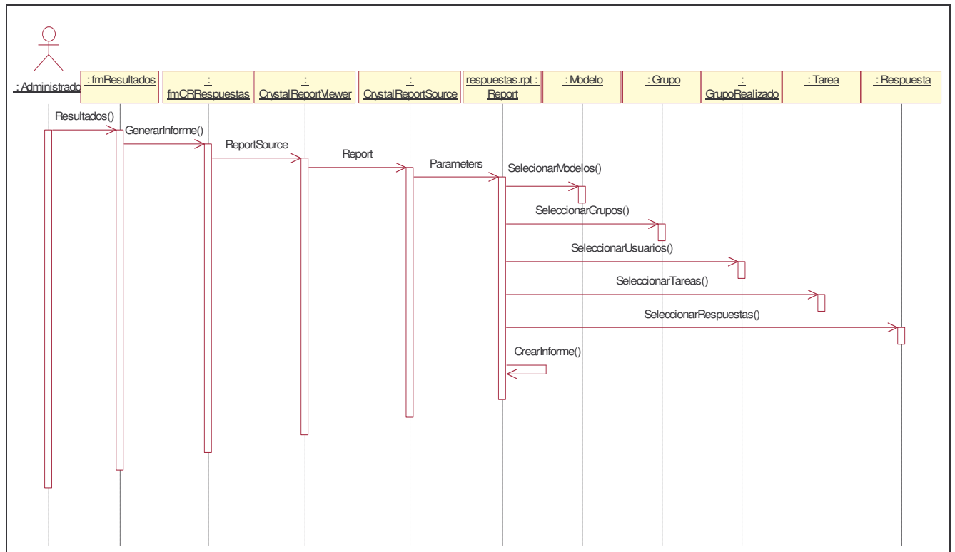
Figura A.24. Diagrama de Secuencia del caso de uso Visualizar Respuestas
