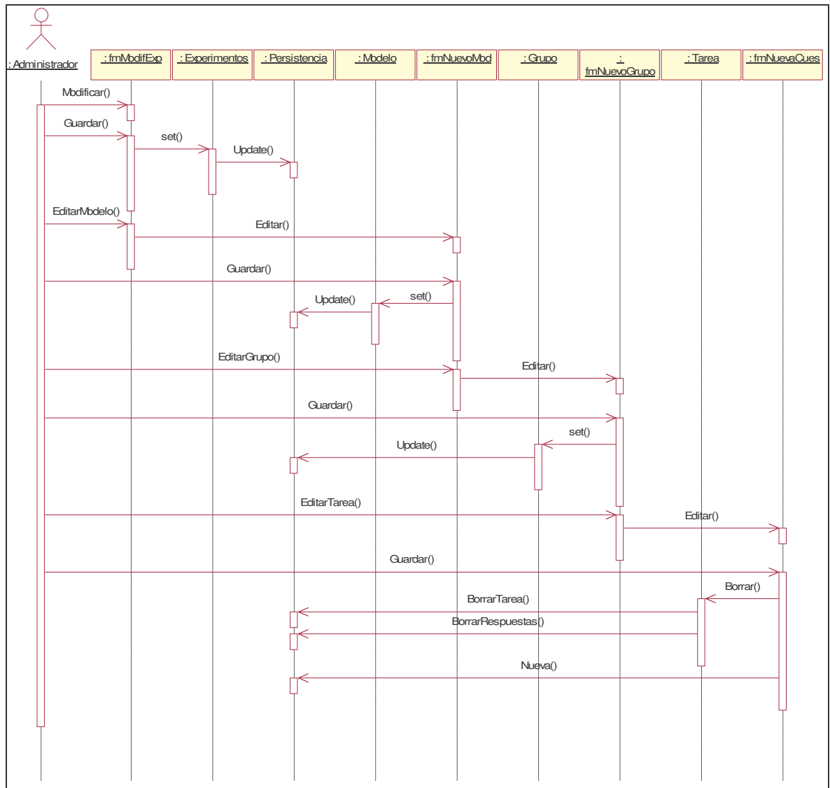
Figura A.12. Diagrama de Secuencia del caso de uso Modificar Encuesta o Experimento
