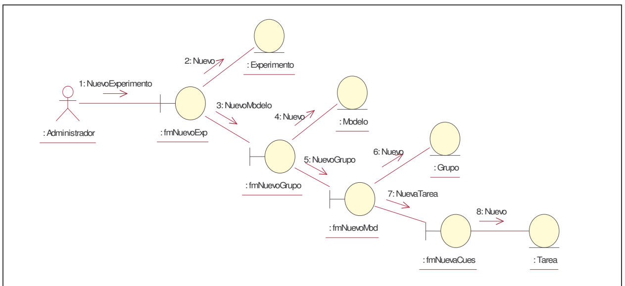
Figura 5.4. Interacción de las clases para el caso de uso Definir Encuesta o Experimento
