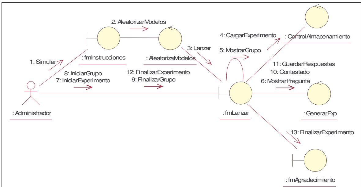
Figura 5.8. Interacción de las clases para el caso de uso Realizar Encuesta o Experimento
