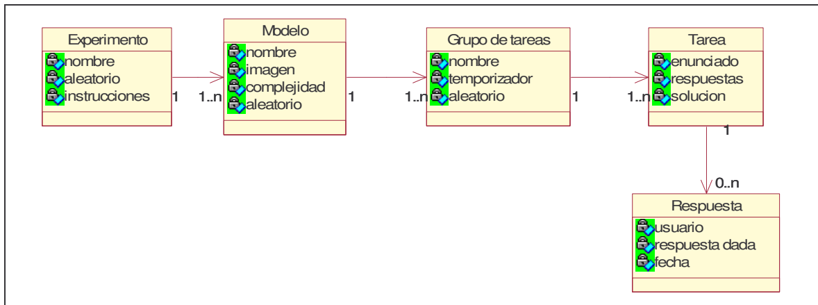
Figura 5.1. Modelo del Dominio
