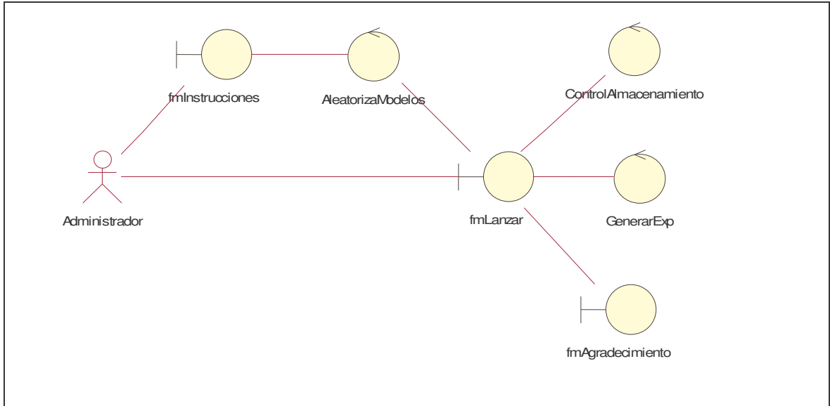
Figura 5.7. Clases del caso de uso-análisis Realizar Encuesta o Experimento
