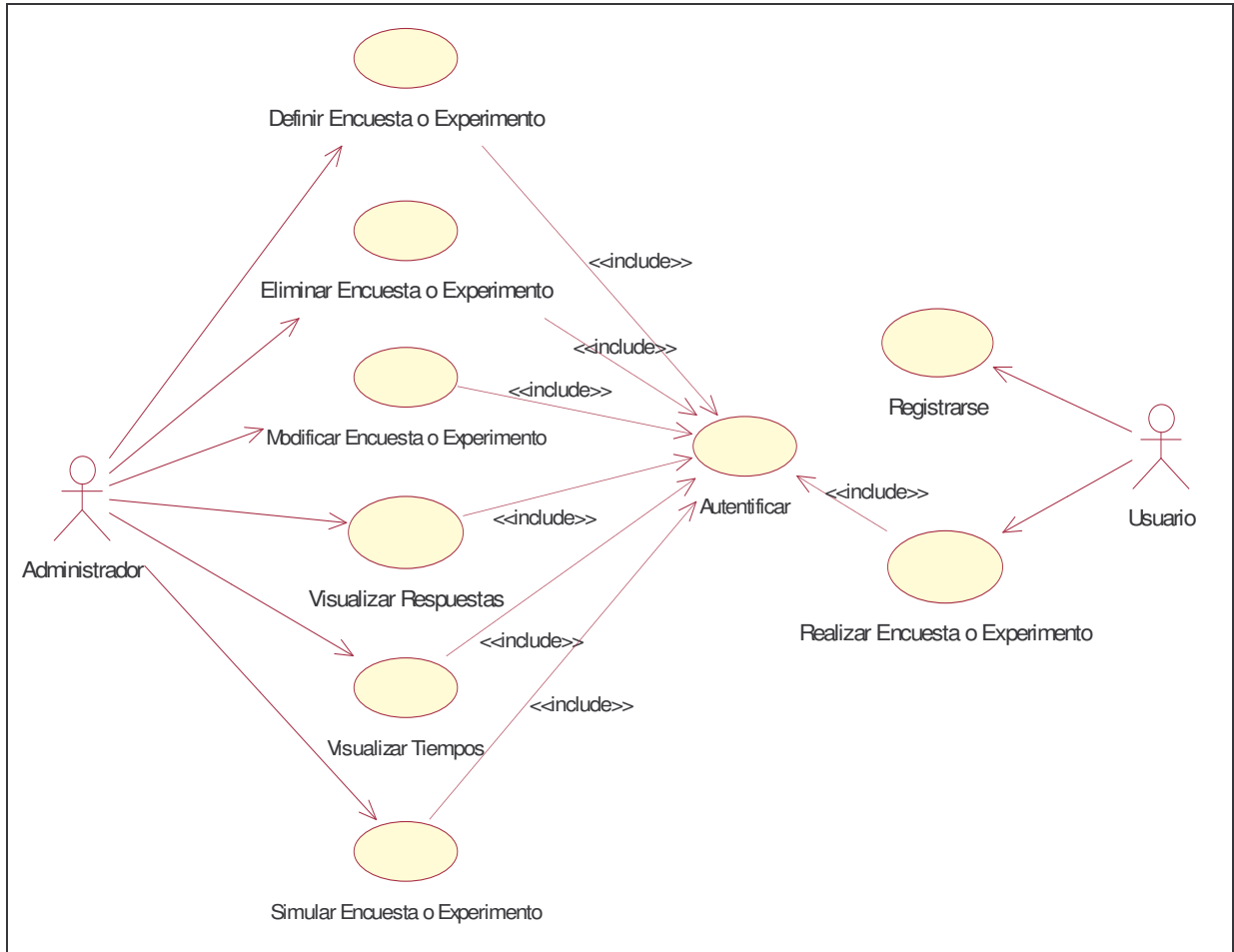
Figura 5.2. Modelo de casos de uso
