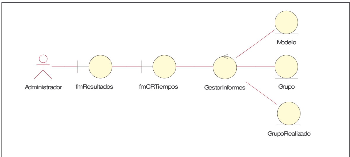
Figura 5.5. Clases del caso de uso Visualizar Tiempos
