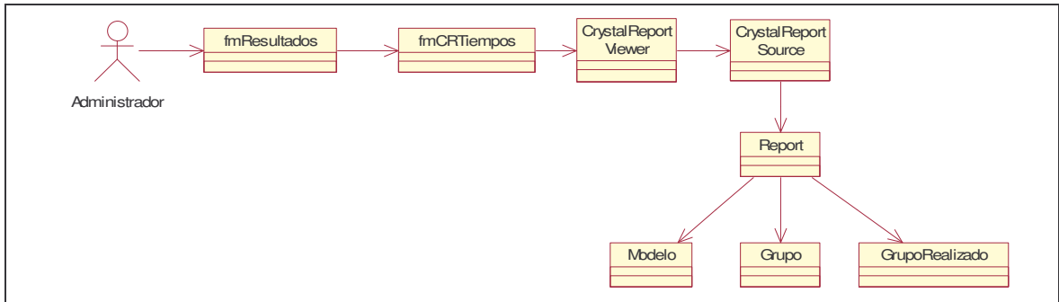
Figura 5.11. Clases del caso de uso-diseño Visualizar Tiempos
