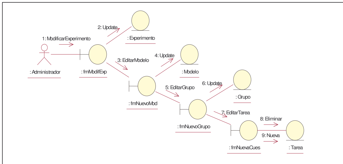
Figura A.10. Interacción de las clases para el caso de uso Modificar Encuesta o Experimento
