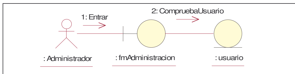
Figura A.2. Interacción de las clases para el caso de uso Autenticar
