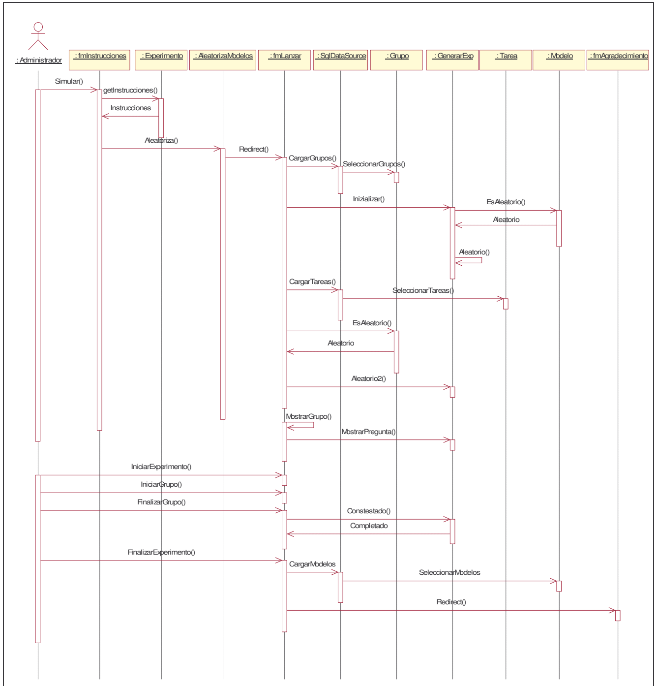
Figura A.20. Diagrama de Secuencia del caso de uso Simular Encuesta o Experimento
