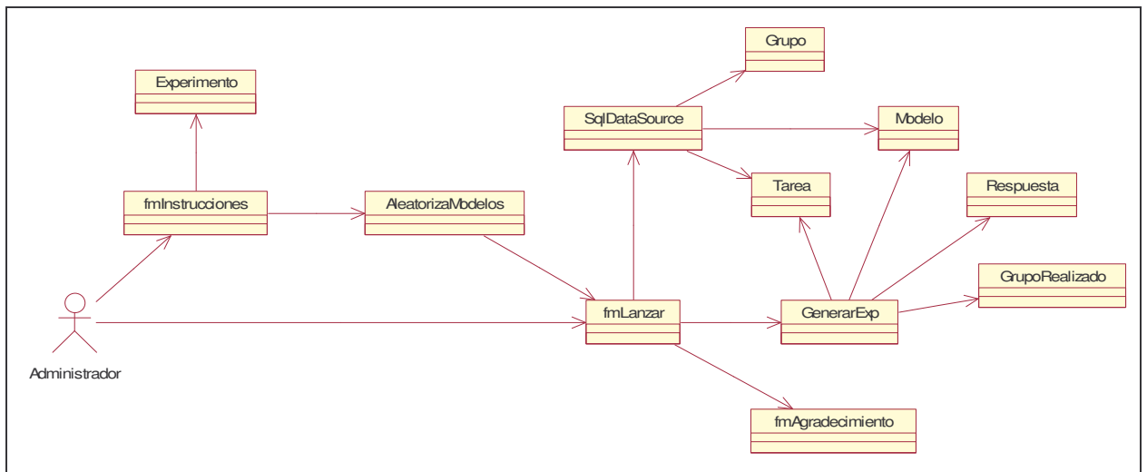
Figura 5.13. Clases del caso de uso-diseño Realizar Encuesta o Experimento
