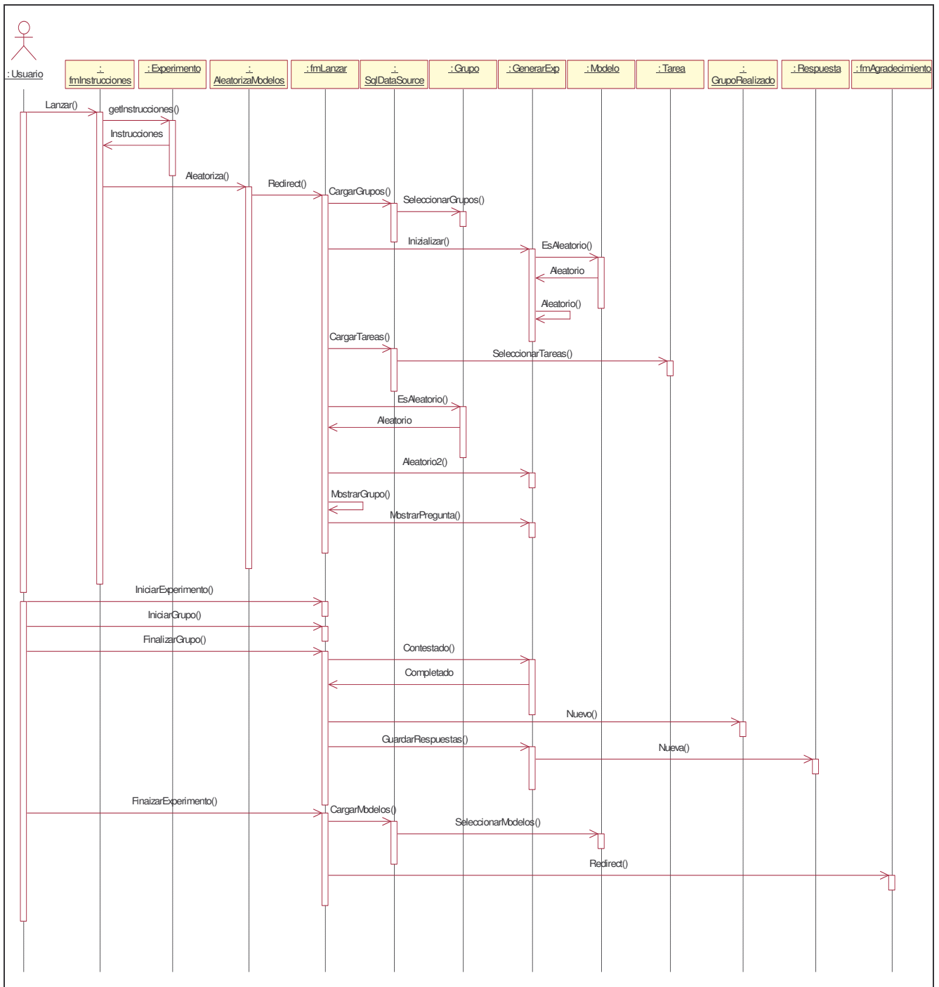
Figura 5.14. Diagrama de Secuencia del caso de uso Realizar Encuesta o Experimento
