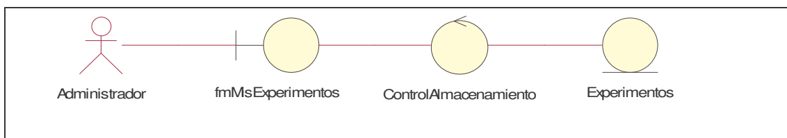
Figura A.13. Clases del caso de uso-análisis Eliminar Encuesta o Experimento
