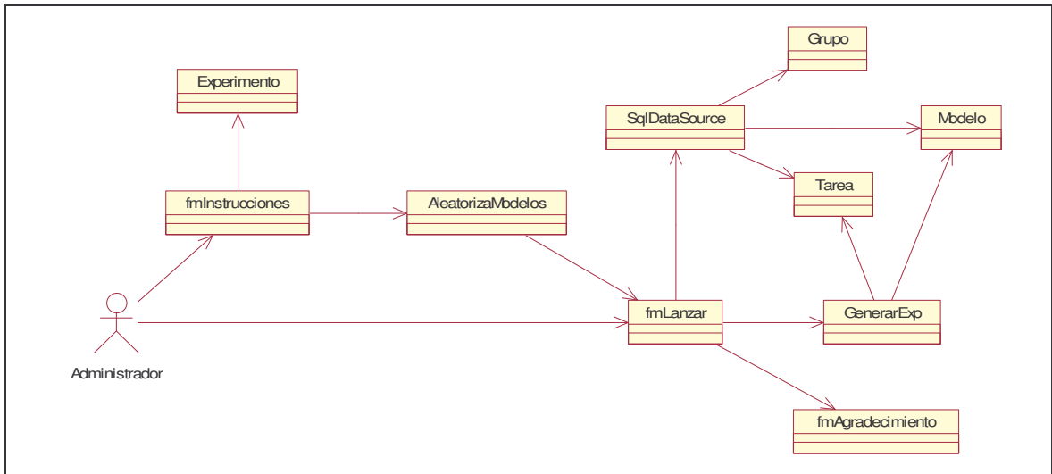
Figura A.19. Clases del caso de uso-diseño Simular Encuesta o Experimento
