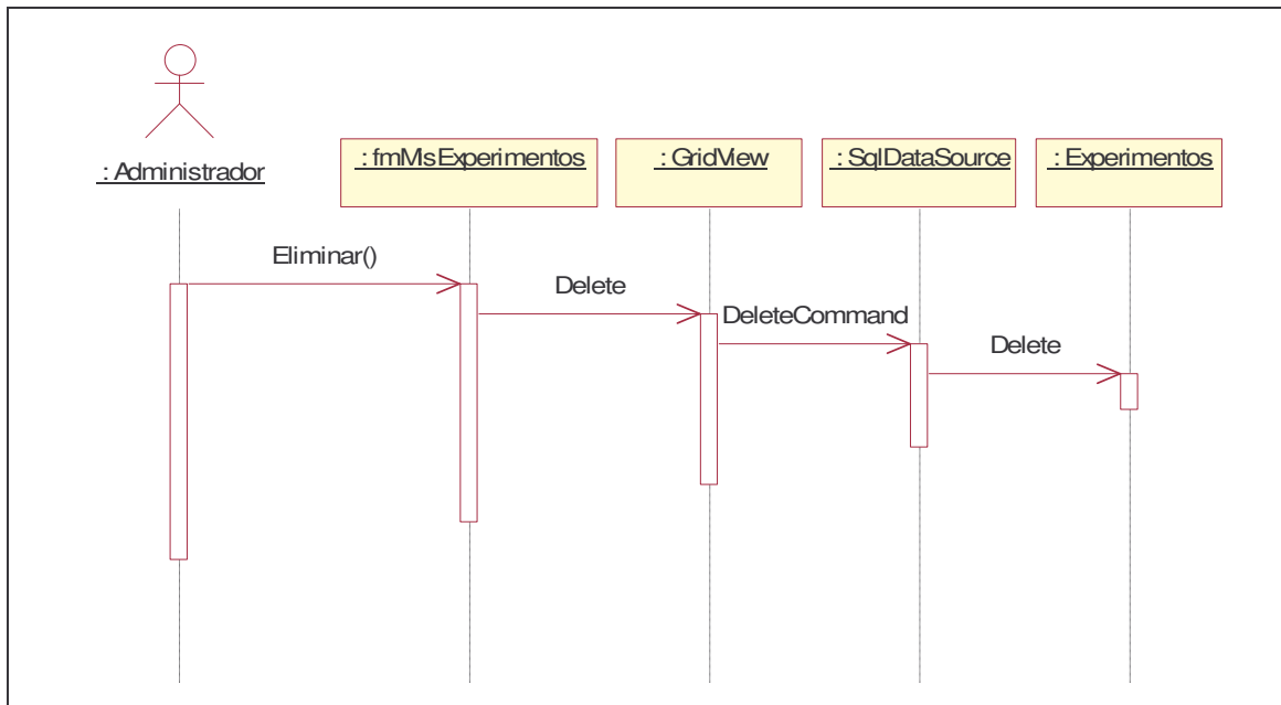
Figura A.16. Diagrama de Secuencia del caso de uso Eliminar Encuesta o Experimento
