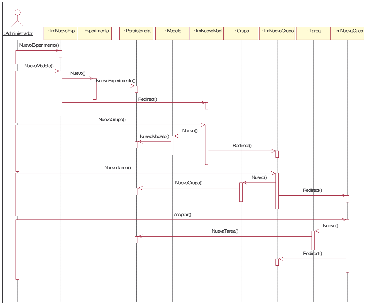
Figura 5.10. Diagrama de Secuencia del caso de uso Definir Encuesta o Experimento
