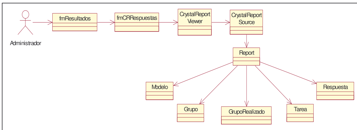
Figura A.23. Clases del caso de uso-diseño Visualizar Respuestas
