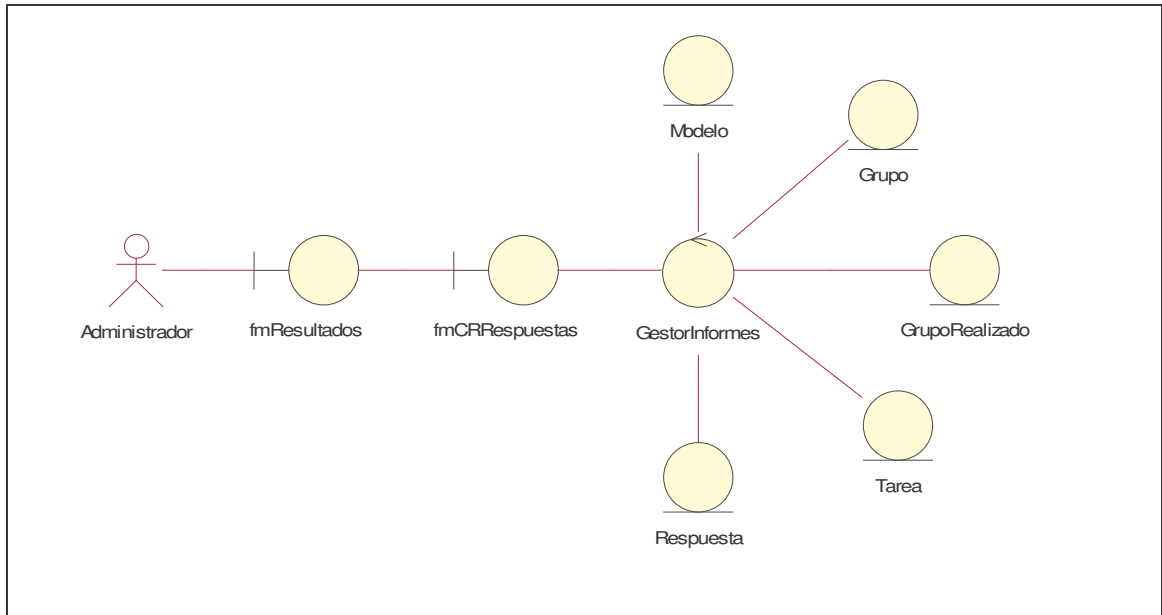
Figura A.21. Clases del caso de uso Visualizar Respuestas
