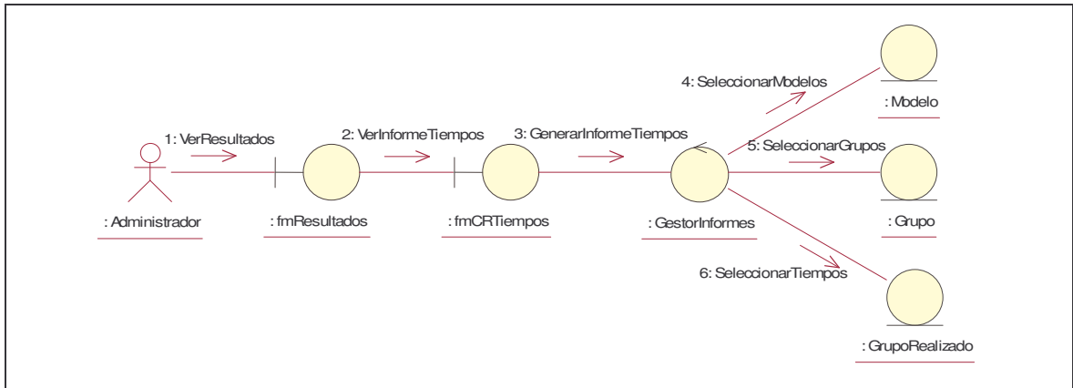
Figura 5.6. Interacción de las clases para el caso de uso Visualizar Tiempos
