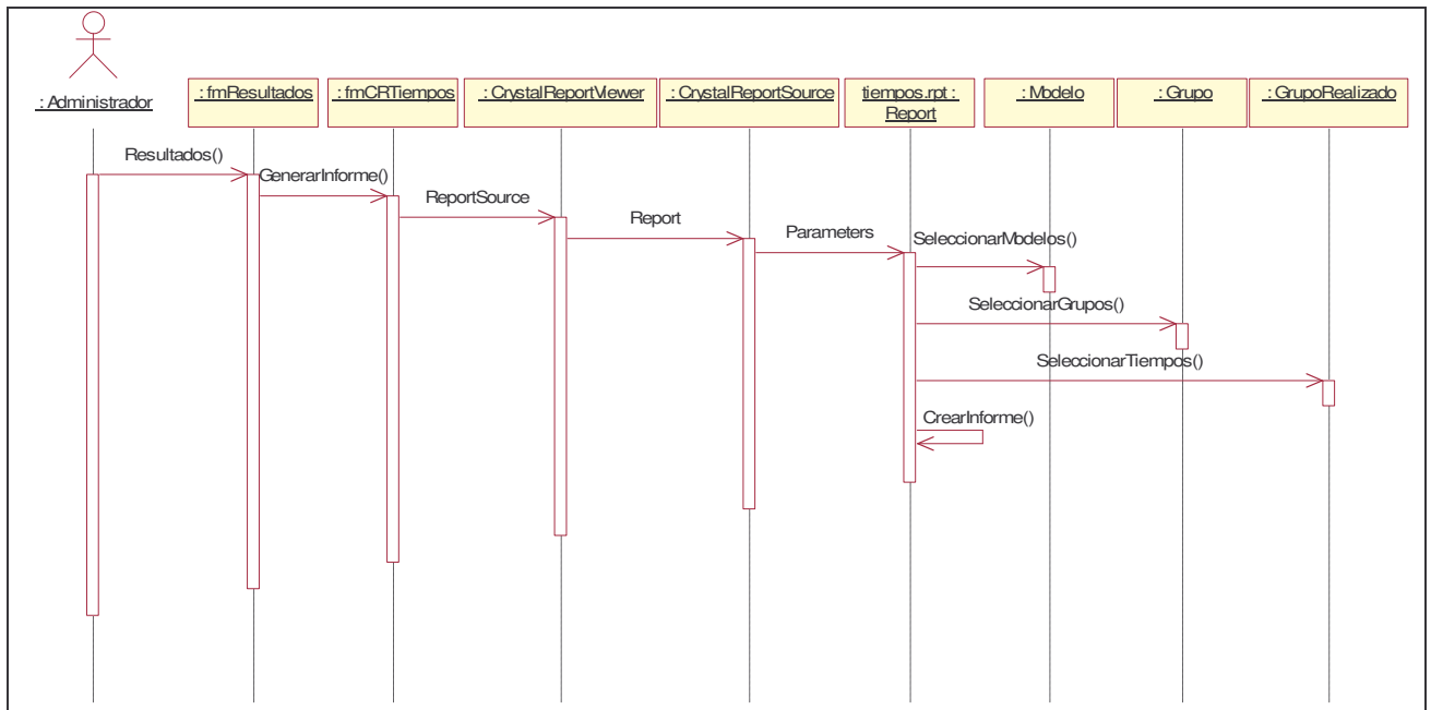
Figura 5.12. Diagrama de Secuencia del caso de uso Visualizar Tiempos
