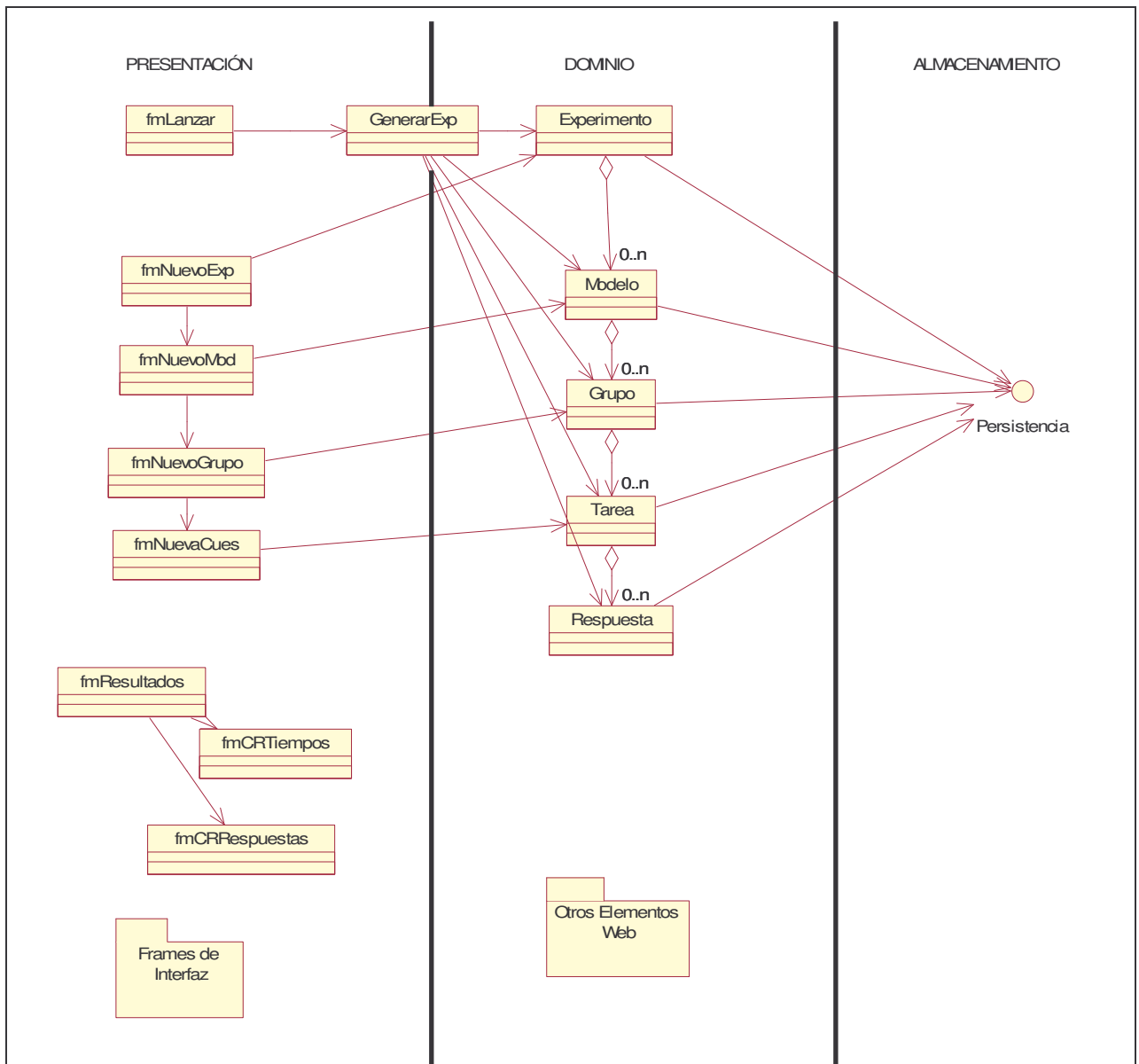
Figura 5.15. Arquitectura en Tres Capas de la Aplicación
