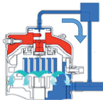
Válvula de alivio de presión abierta (descarga a la succión)
